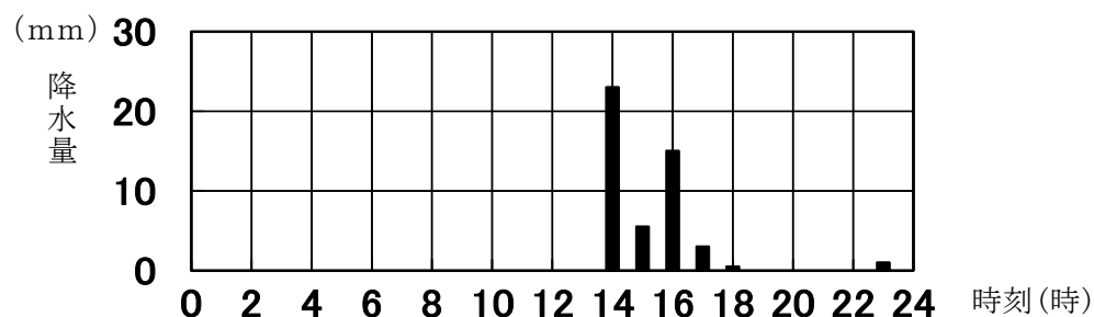
図4 1時間ごとの降水量の変化
